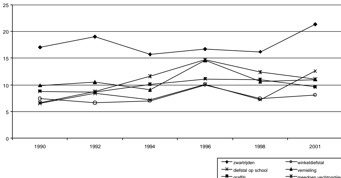
Figuur 1: Ontwikkeling van het percentage delictplegers, voor enkele veel voor komende feiten, in %
