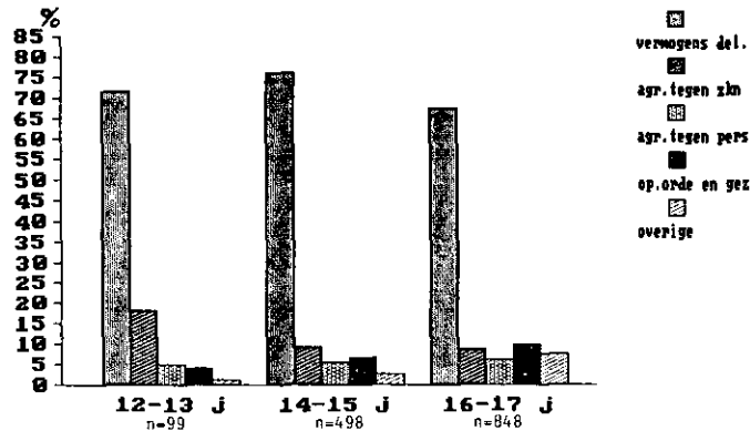
Figuur 18: Delicttype en leeftijd (in %; n=1.445)
